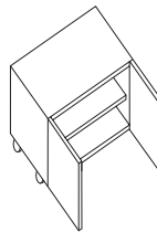
D79CM Double door H635 x W600 x D600
